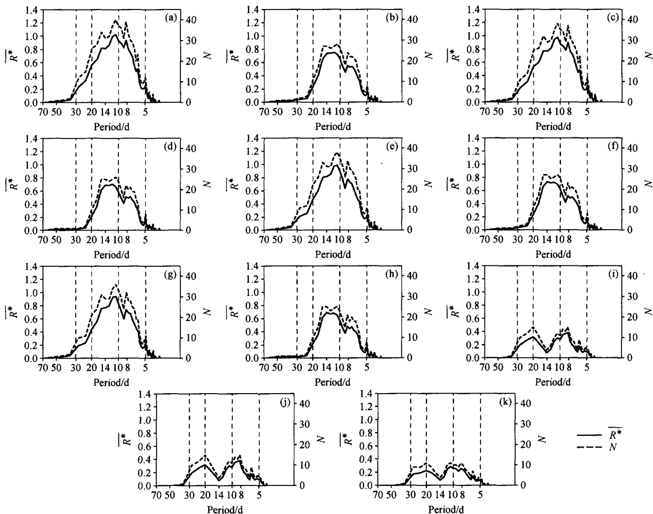
图5 1948~2005年NAMI全年(365天)标准化功率谱 \overline{R^*} 合成及对应周期上功率谱通过显著性检验的年份总数统计 N : (a) 所有年份; (b) 所有不含准3 W的年份; (c) 所有含准1 W的年份; (d) 含准1 W、无准3 W的年份; (e) 所有含准2 W的年份; (f) 含准2 W、无准3 W的年份; (g) 既有准1 W又有准2 W的所有年份; (h) 既有准1 W又有准2 W年份, 但无准3 W的年份; (i) 含有准3 W的所有年份; (j) 既有准1 W又有准3 W的所有年份; (k) 既有准2 W又有准3 W的所有年份
