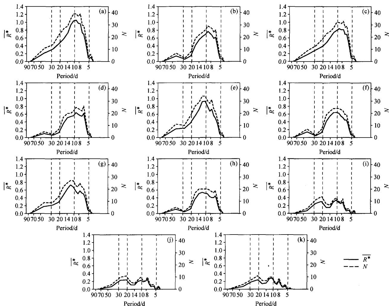
图9 同图5, 但为 SAMI 前半年 (1~6 月)
