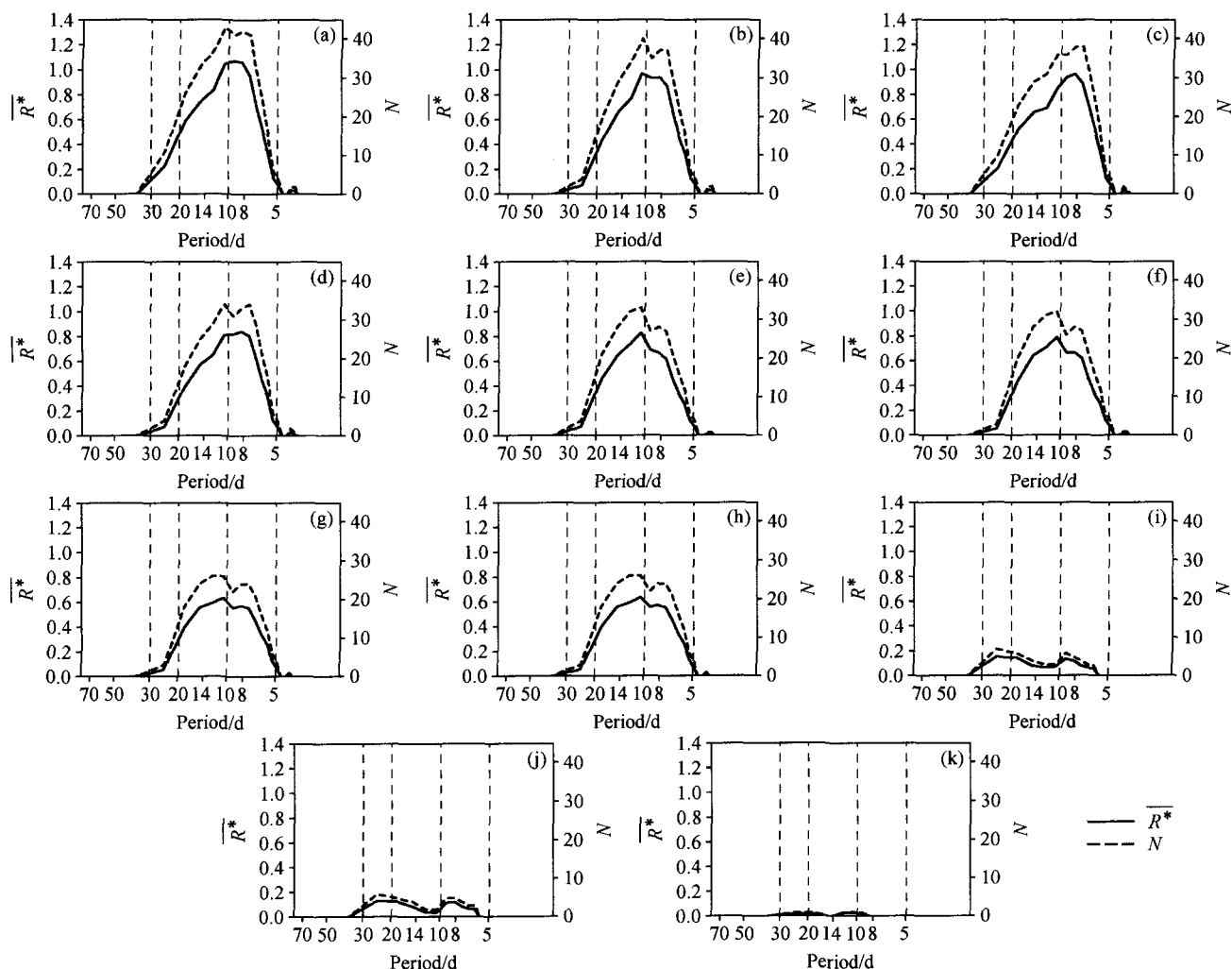
图7 同图5, 但为NAMI非活跃期(5~9月)
