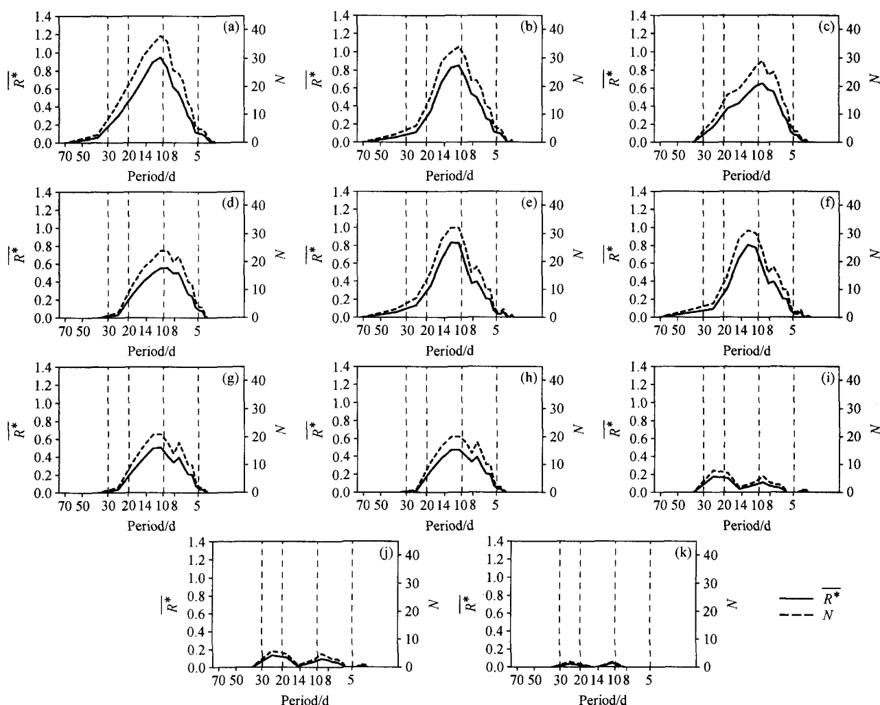
图6 同图5, 但为MAMI活跃期(11~3月)
