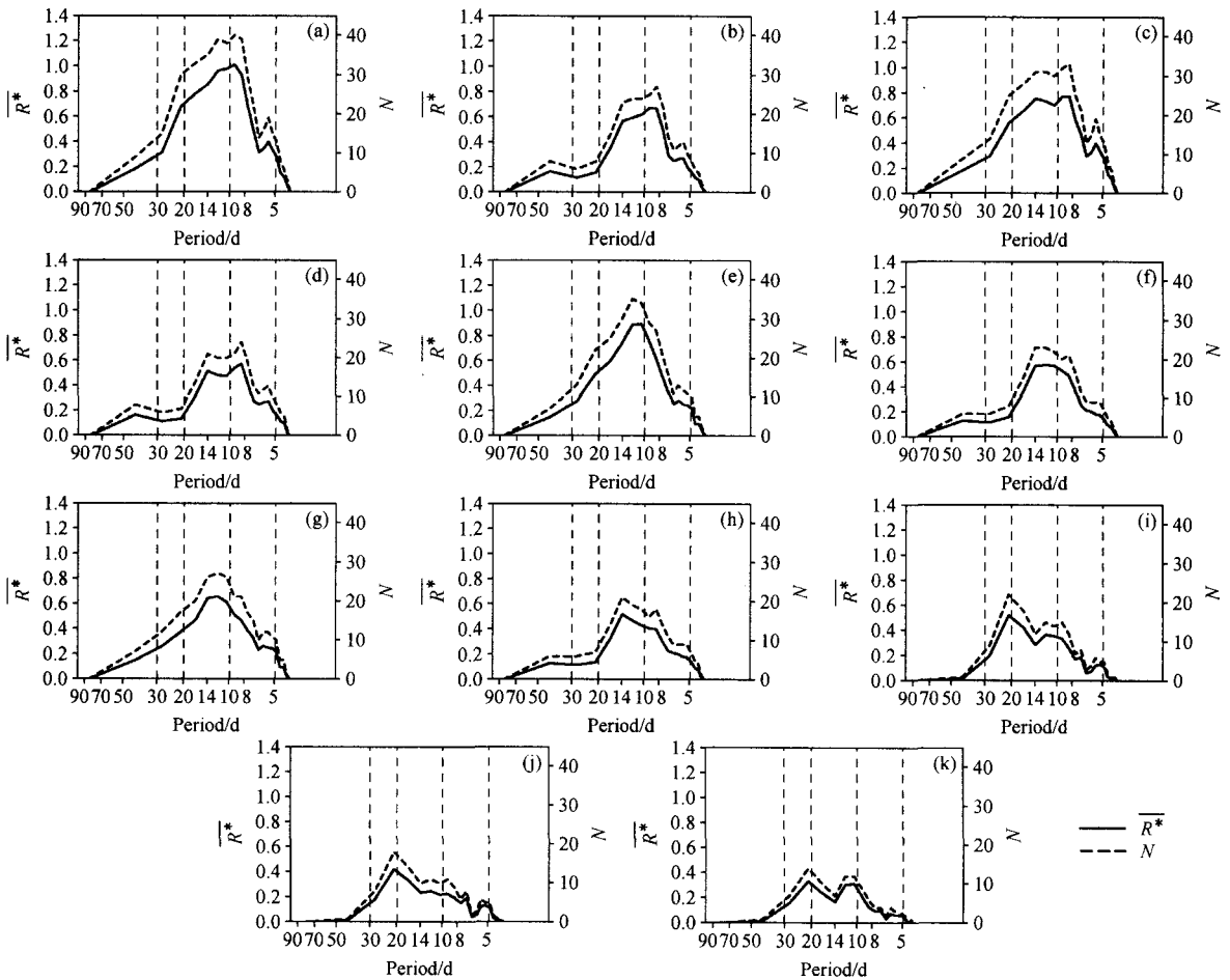
图 10 同图 5, 但为 SAMI 后半半年 (7~12 月)
