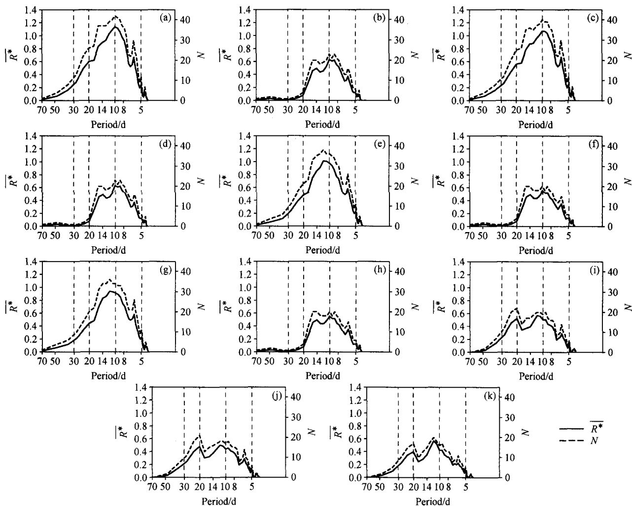
图8 同图5, 但为 SAMI 全年 (365 天)
