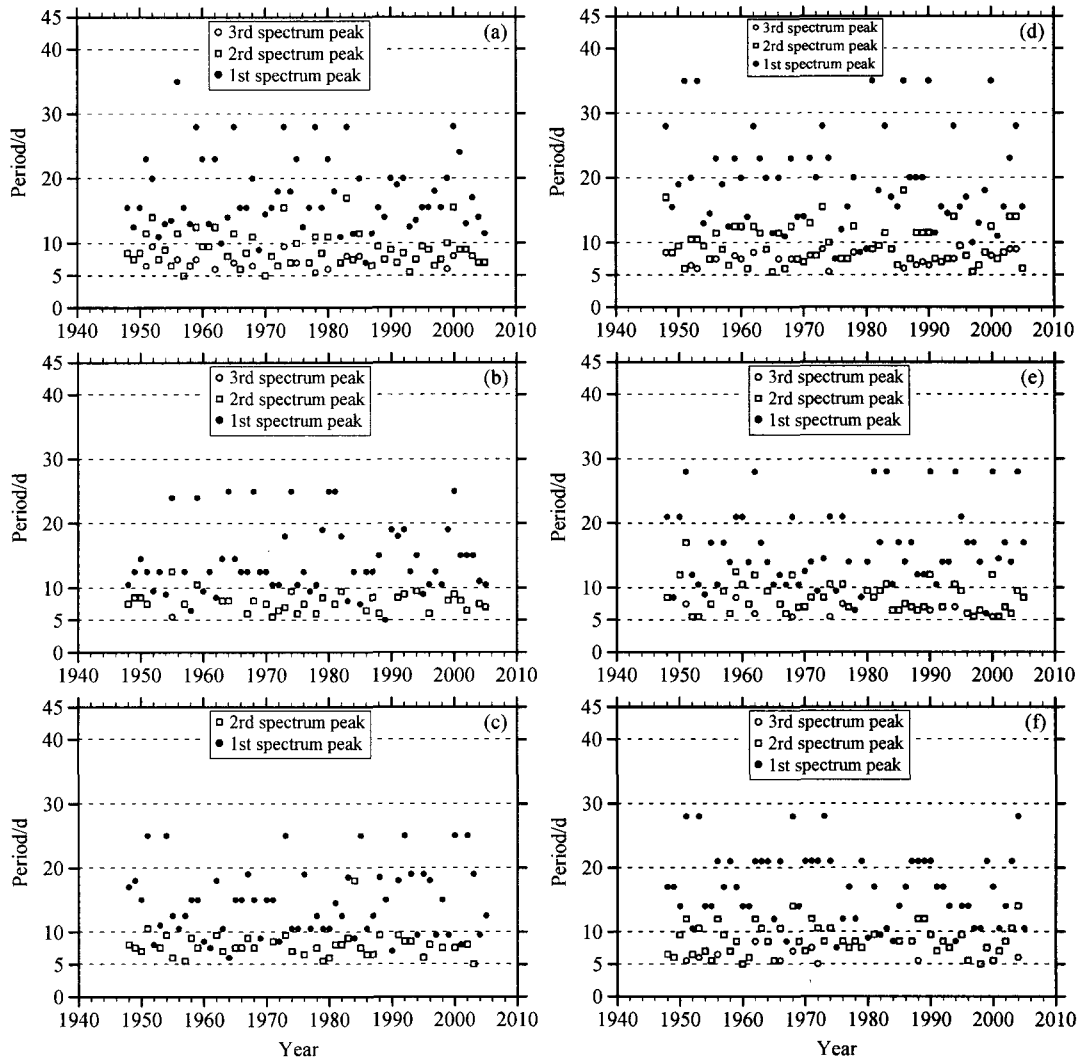
图4 1948~2005年功率谱分析显著谱峰对应的周期分布: (a) NAMI全年; (b) NAMI活跃期; (c) NAMI非活跃期; (d) SAMI全年; (e) SAMI前半年; (f) SAMI后半年
