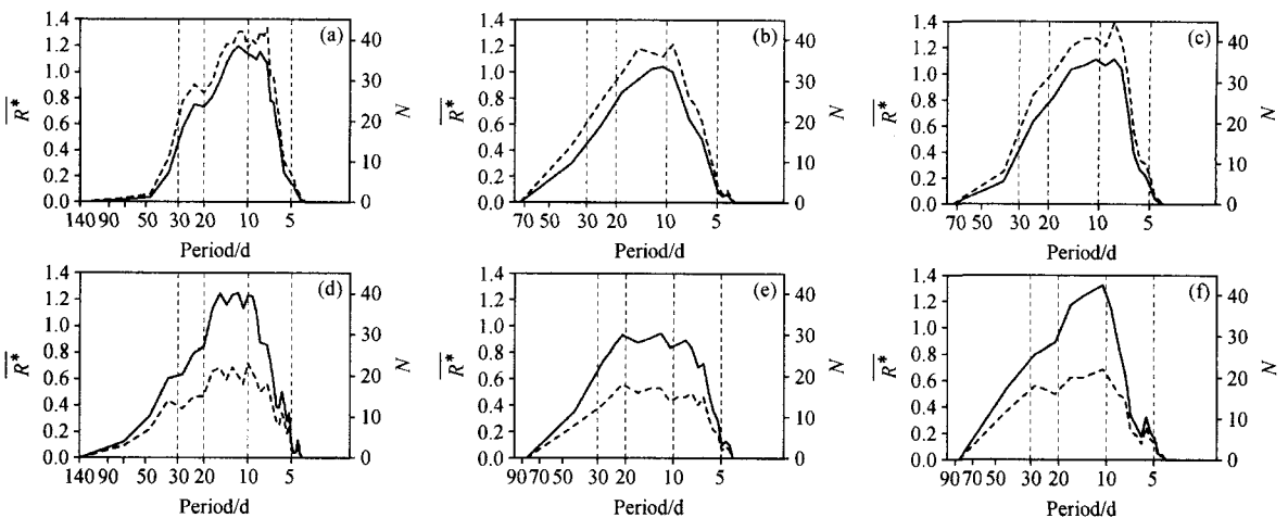
图 11 CPC-NAMI (1950~2005 年) (a) 全年、(b) 活跃期、(c) 非活跃期和 CPC-SAMI (1979~2005 年) (d) 全年、(e) 前半、(f) 后半 年标准化功率谱 \overline{R^*} 合成及对应周期上功率谱通过显著性检验的年份总数统计 N
