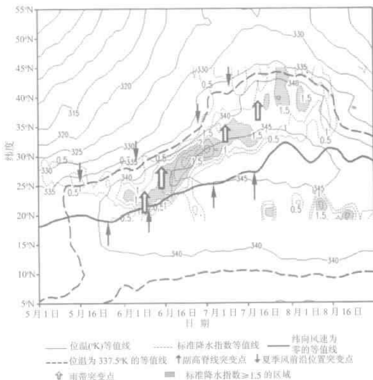
图 4 1951~2000 年平均 5~8 月 850 hPa 上 110~120°E 5 天滑动平均位温
