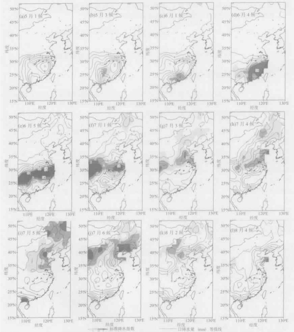
图 3 5~8月代表候平均日降水量 R_5 (实线)、标准降水指数 S_R (阴影) 气候值的分布图
