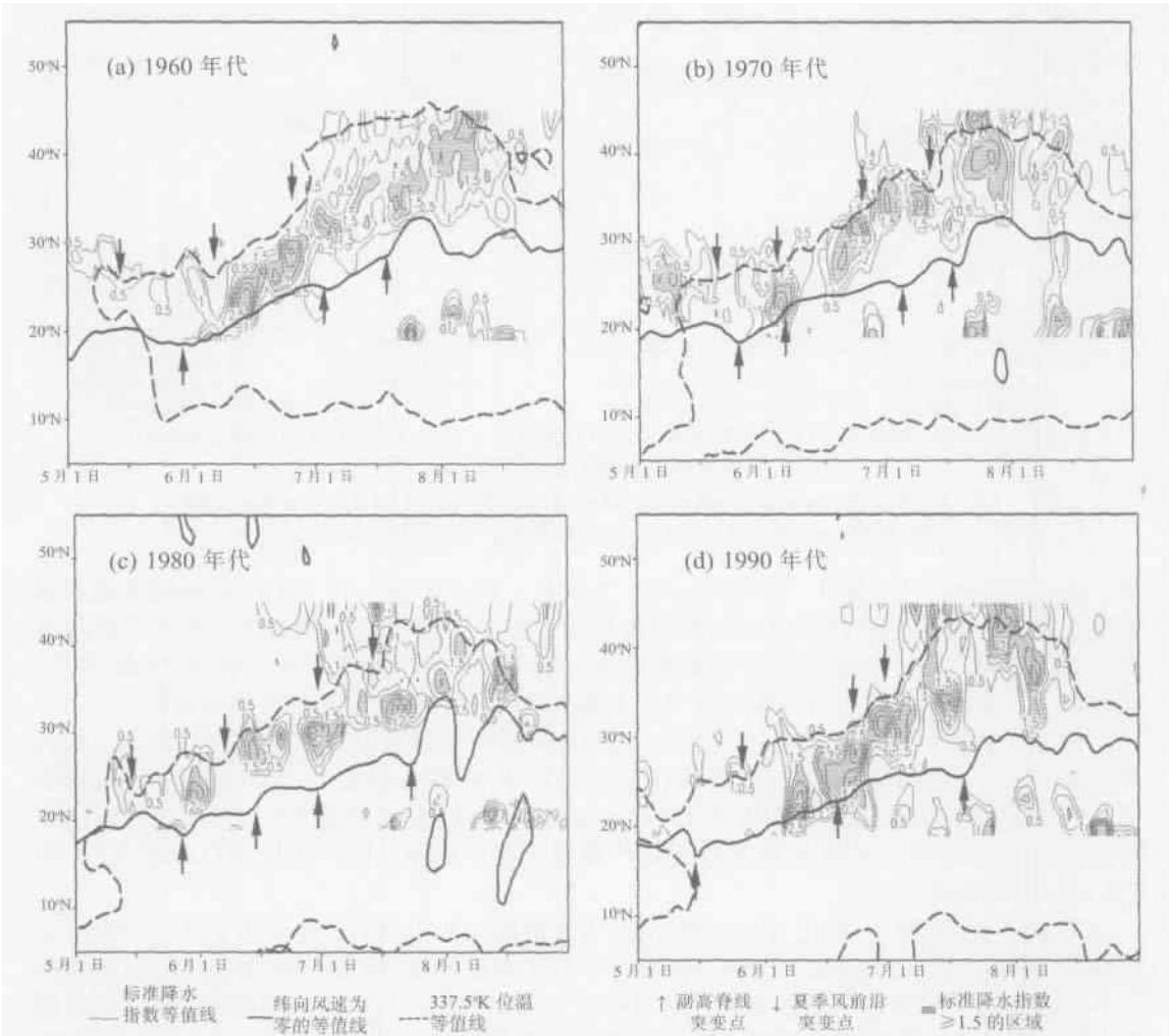
图 5 各年代 5~8 月 110~120°E 陆地 5 天滑动平均标准降水指数 S_r (实线)、850 hPa 上 110~120°E 5 天滑动平均 \theta_{337.5} = 337.5^\circ\text{K} 特征线、500 hPa 上 125~145°E 5 天滑动平均 u = 0 线的时间 - 纬度剖面图
