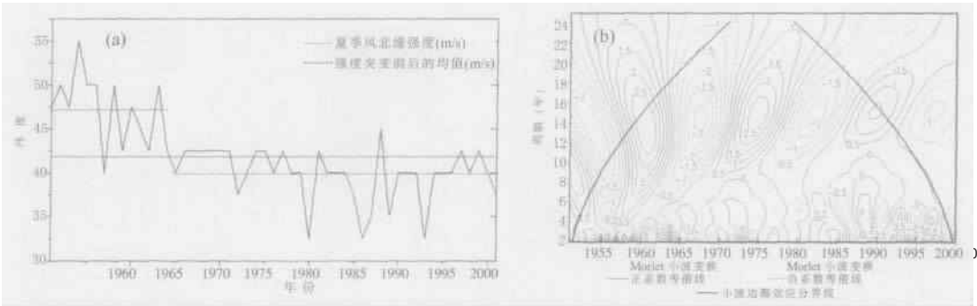
图 9 1951~2001 年 110~120°E 夏季风北界强度的时间变化曲线(a), Morlet 小波变换系数分布(b) Fig. 9 The same as Figure 8 except for the north edge intensity
