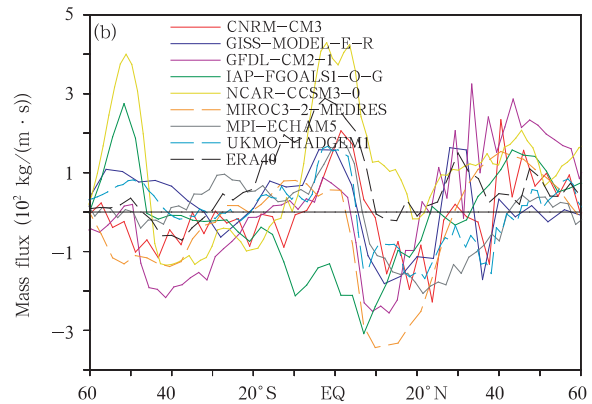
图3 AMIP全球大气环流模式模拟的和观测的7月(a)、1月(b)和年平均(c)的纬向平均(60°N—60°S)大气经向质量通量 \bar{I} 的经向分布
