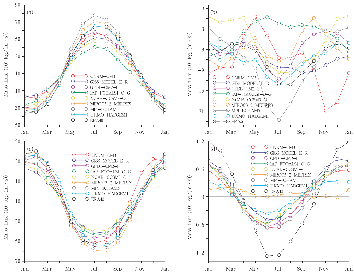
图 2 AMIP 全球大气环流模式模拟的和观测的赤道上纬向平均的分层质量通量的年循环
