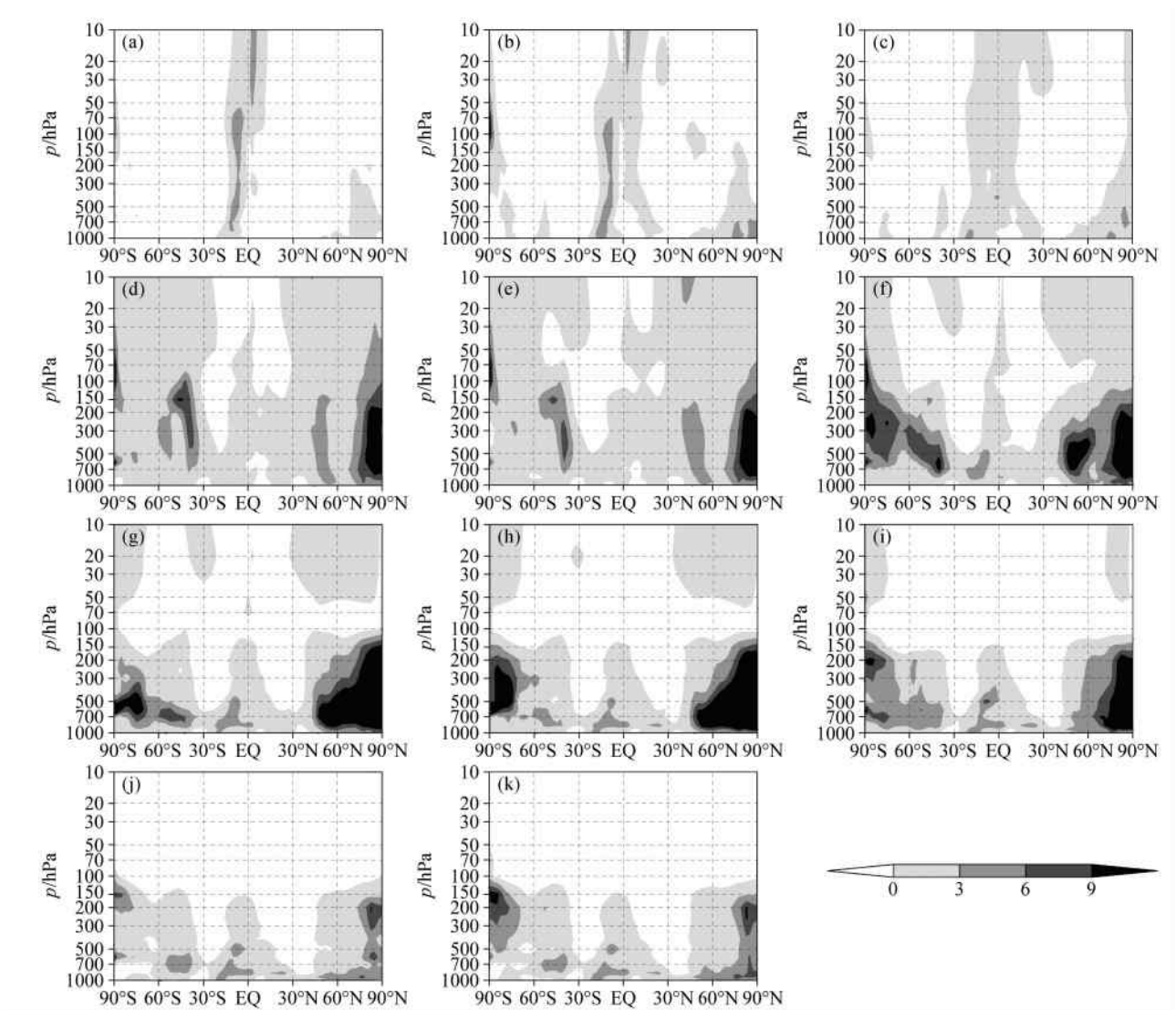
图 8 风场季节变化相对于地球自转速度下相对大小的纬向平均分布 (阴影): (a-k) 自转周期为地球自转周期的 1/10、1/5、1/3、2 倍、2.5 倍、5 倍、10 倍、16 倍、50 倍、150 倍、243 倍 Fig. 8 Zonal-mean relative seasonal change of wind for different rotation periods compared to the Earth rotation period ( \hat{\delta}_\Omega ): (a) 1/10 d; (b) 1/5 d; (c) 1/3 d; (d) 2 d; (e) 2.5 d; (f) 5 d; (g) 10 d; (h) 16 d; (i) 50 d; (j) 150 d; (k) 243 d
