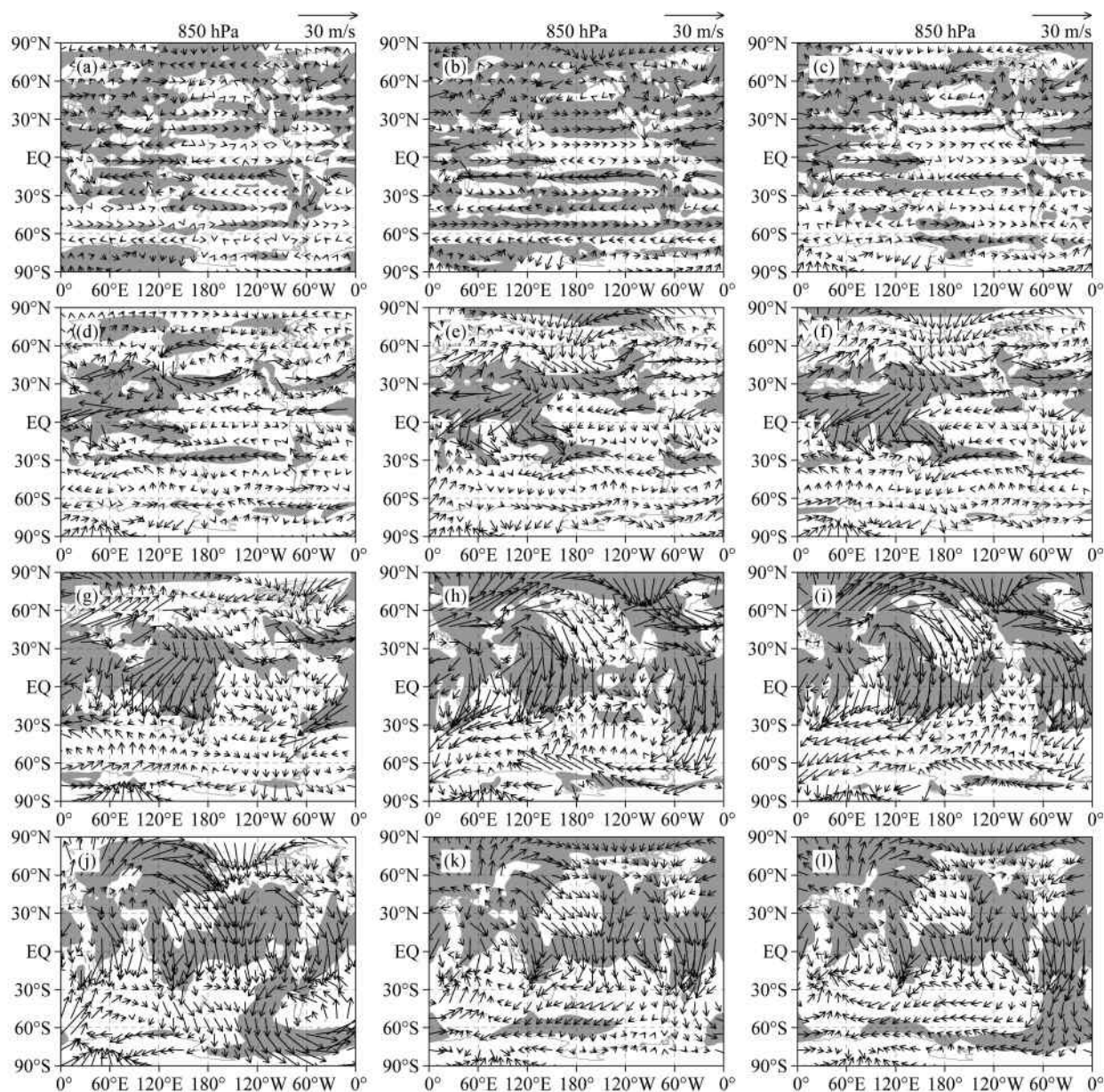
图1 850 hPa高度的1月、7月风场差和季风区(阴影)的全球分布:(a-l)自转周期为地球自转周期的1/10、1/5、1/3、1倍、2倍、2.5倍、5倍、10倍、16倍、50倍、150倍、243倍
