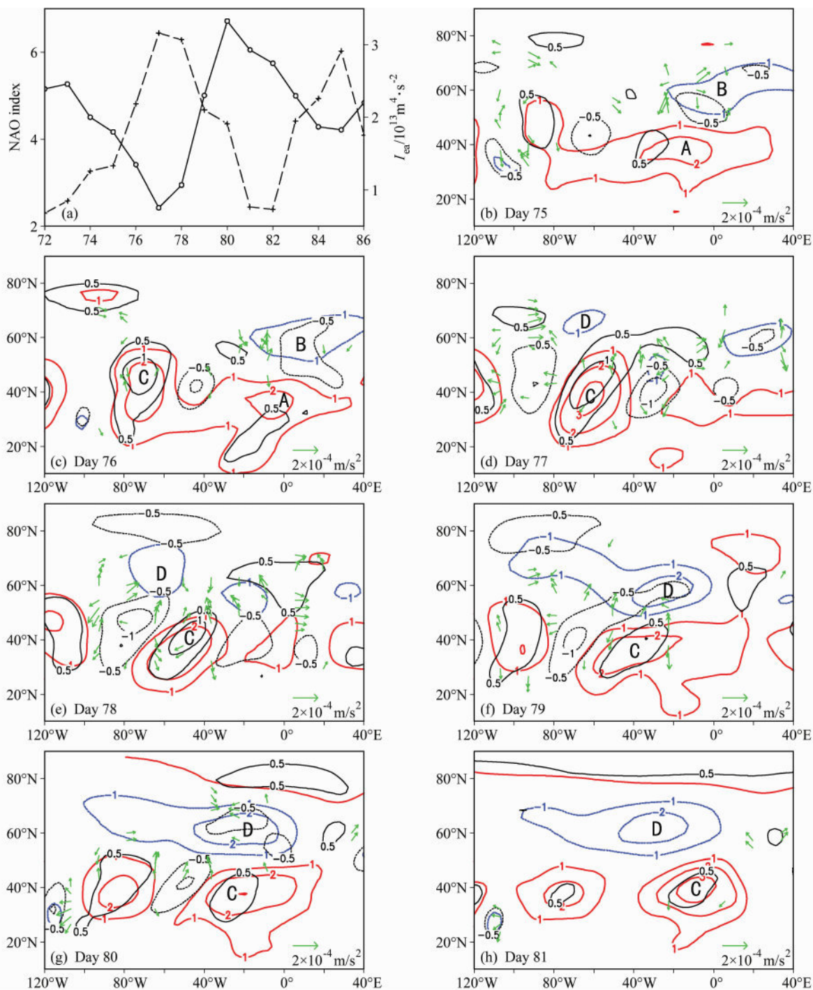
图4 (a) 同图3, 但为1996/1997年冬季第72~86天; (b-h) 第75~81天的低频环流 \bar{\psi}^a (彩色等值线, 单位: 10^7 \text{ m}^2/\text{s} )、瞬变涡旋 \psi' (黑色等值线, 单位: 10^7 \text{ m}^2/\text{s} )以及瞬变涡度通量 \mathbf{F} (绿色矢量)。A-D: 低频异常
