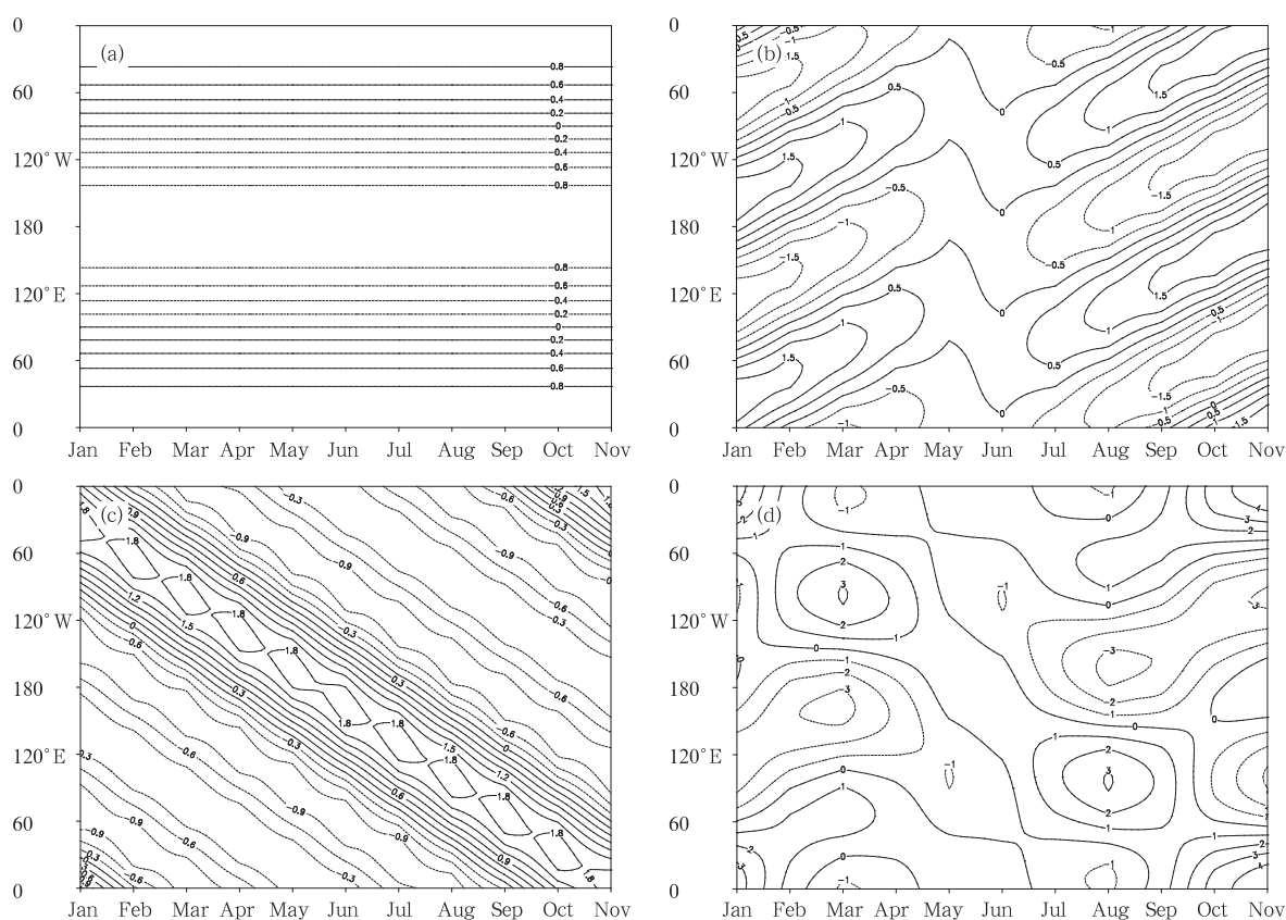
图6 理想函数构造的具有双向传播特征的时-空序列 F_2(x, t) 经过时-空二维波传播分解后得到的各分量的时-空分布, 以及由各分量再次合成得到的时-空序列的时-空分布
