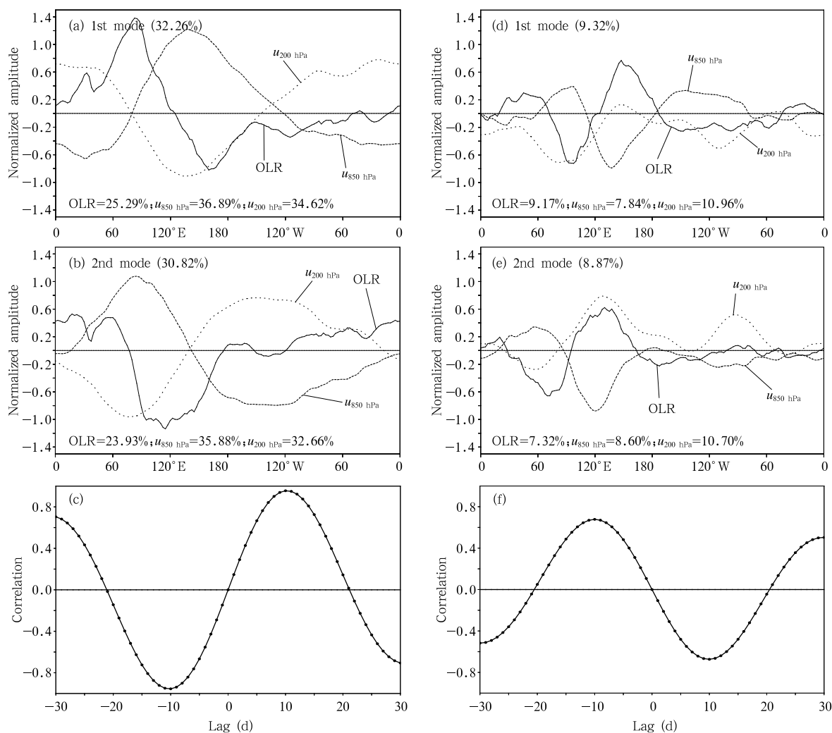
图 8 OLR、850 和 200 hPa 纬向风 3 个变量东传和西传分量 30—60 d 滤波且 15°S—15°N 平均之后,
