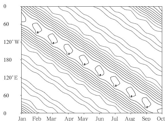
图 1 理想函数构造的具有单向传播特征的时-空序列 f(x, t) 的时-空分布
