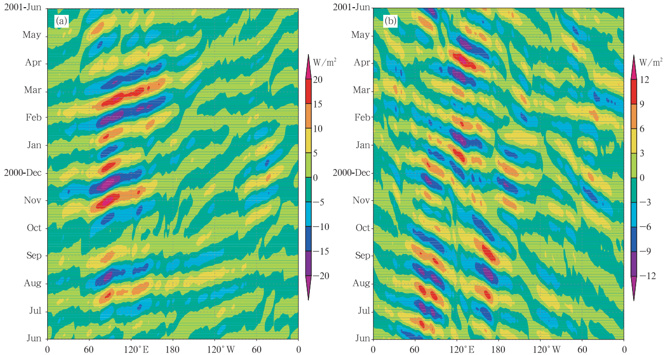
图 9 2000 年 6 月—2001 年 6 月,OLR 东传(a)和西传分量(b)的经度-时间剖面(单位: \text{W/m}^2 )
