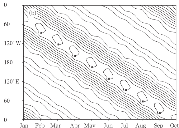
图 4 理想函数构造的具有双向传播特征的时-空序列 F_1(x, t) 经过时-空二维波传播分解后得到的东传分量、西传分量以及由东传分量和西传分量合成的时-空序列的时-空分布
