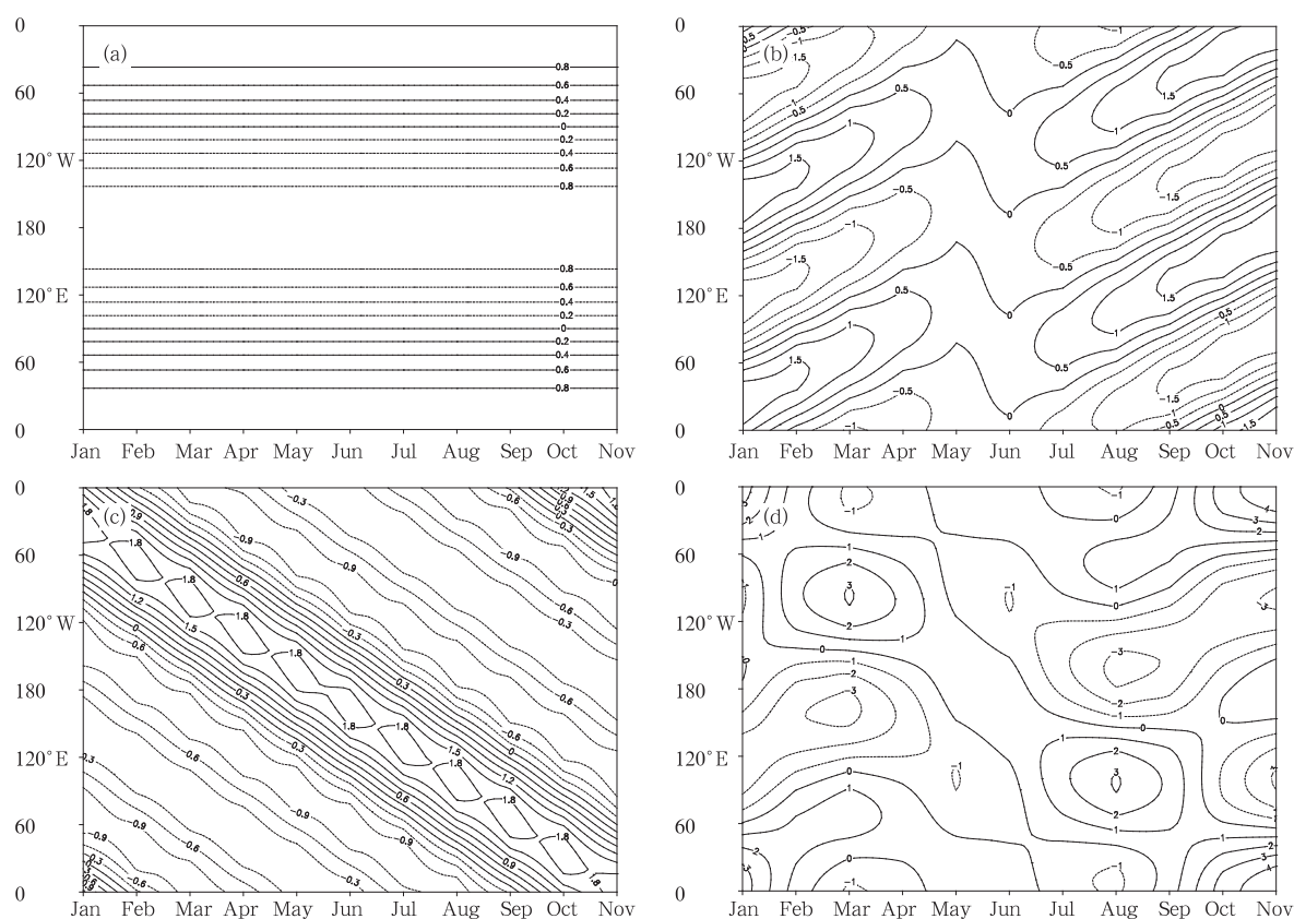
图5 理想函数构造的具有双向传播特征的时-空序列 F_2(x, t) 的时-空分布,
