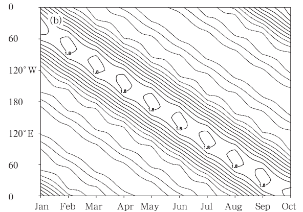
图 3 理想函数构造的具有双向传播特征的时-空序列 F_1(x, t) 的时-空分布, 以及合成 F_1(x, t) 的两部分具有不同传播方向的分量 f_1(x, t) 和 f_2(x, t) 的时-空分布 (a. 向东传播的分量 f_2(x, t) , b. 向西传播的分量 f_1(x, t) , c. 时-空序列 F_1(x, t) )
