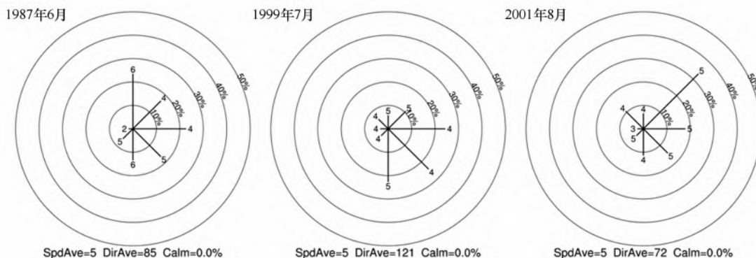
图3 1987年6月(左),1999年7月(中)和2001年8月(右),模拟区域的风向玫瑰图;其他同图2
