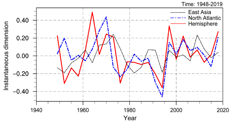
图7 1948~2019年东亚—西北太平洋(20°~60°N, 90°E~150°W)、北大西洋(22°~70°N, 80°W~50°E)和北半球区域(0°~90°N)海平面气压的瞬时维度的年代际趋势
