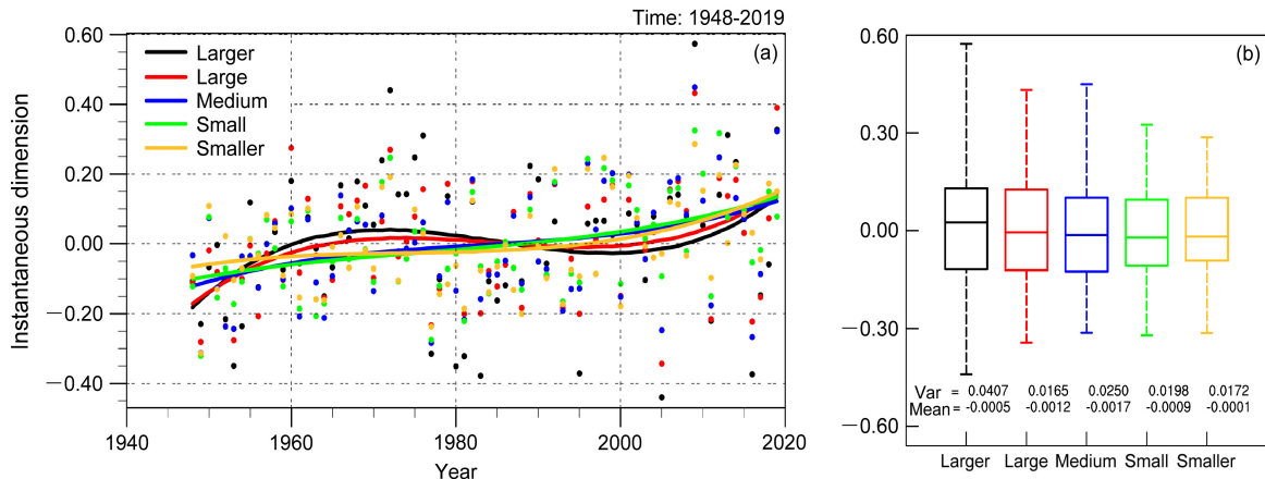
图8 瞬时维度对东亚—西北太平洋海平面气压区域范围选择的敏感性:(a)五个不同大小区域[基于东亚—西北太平洋地区(20°~60°N, 90°E~150°W)的范围,逐次递减5个经度和纬度,产生了5个面积由大到小的区域]海平面气压的逐年瞬时维度值和拟合结果;(b)五个区域瞬时维度的箱线图分布。虚线顶部、底部的短横线、矩形框顶部、底部和中部的横线分别表示瞬时维度的上限、下限、上四分位数、下四分位数和中位数,各区域的方差(Var)和均值(Mean)在图的底部给出
