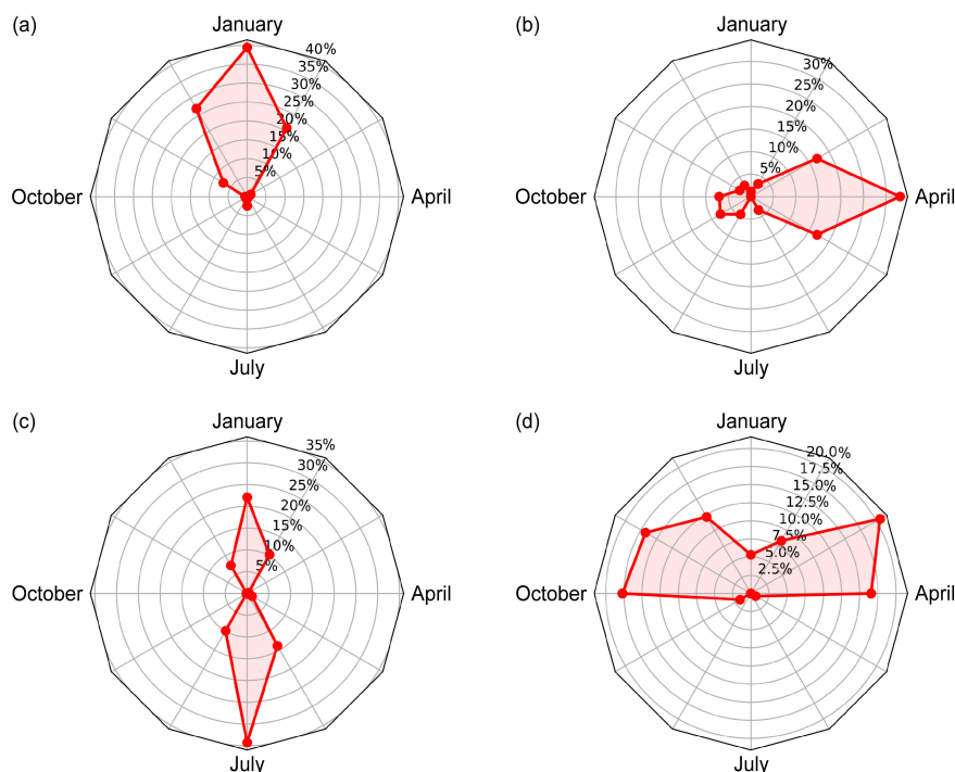
图4 1948~2019年东亚—西北太平洋海平面气压的(a)瞬时维度低值、(b)瞬时维度高值、(c)瞬时稳定度低值、(d)瞬时稳定度高值季节分布。图中圆的12个方向按顺时针顺序分别代表1~12月，同心圆的大小代表该月所占的比例
