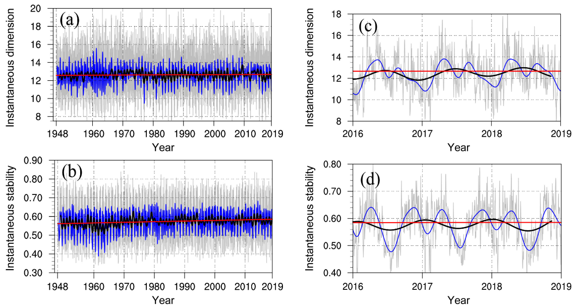
图1 (a、b) 1948~2019年、(c、d) 2016~2019年东亚—西北太平洋海平面气压(a、c)瞬时维度和(b、d)瞬时稳定度的逐日序列(灰线)、3个月低通滤波序列(蓝线)、1年低通滤波序列(黑线)、线性拟合(红线)
