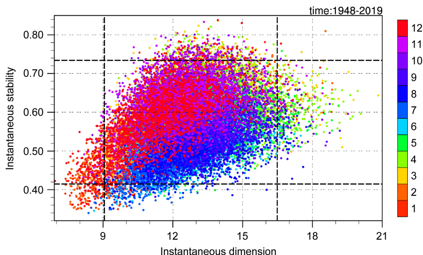
图3 1948~2019年东亚—西北太平洋海平面气压的瞬时维度和瞬时稳定度的散点分布。黑色竖虚线从左至右分别为瞬时维度的0.02和0.98分位数阈值，横虚线从下至上分别为瞬时稳定度的0.02和0.98分位数阈值。点的颜色代表月份
