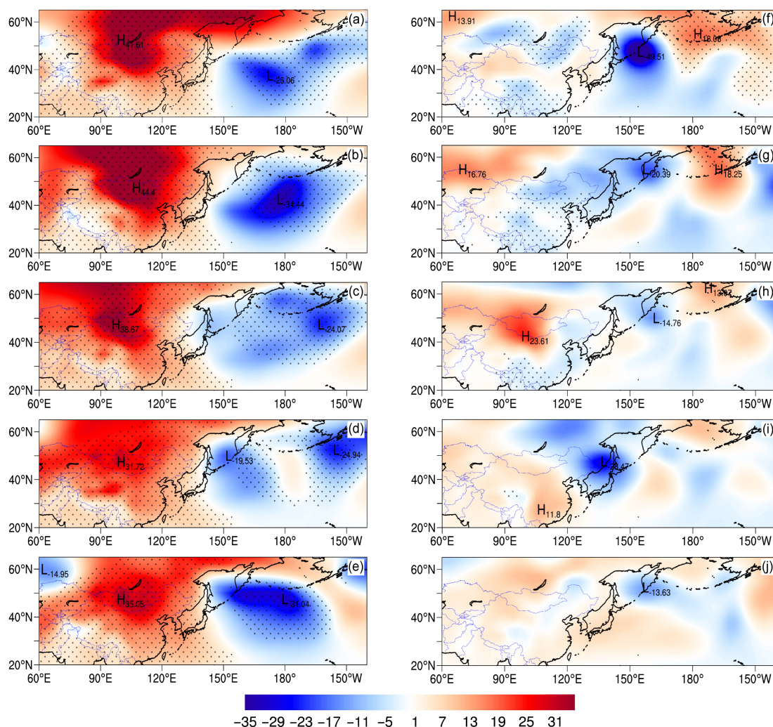
图 6 1948~2019 年东亚—西北太平洋海平面气压的 (a-e) 瞬时维度最低值和 (f-j) 瞬时稳定度最高值对应的 (a, f) 当天、(b, g) 第 2 天、(c, h) 第 4 天、(d, i) 第 6 天和 (e, j) 第 8 天的日平均海平面气压异常场 (单位: hPa) 分布。图中打点区域代表超过 70% 的成员在该区域具有一致的信号分布
