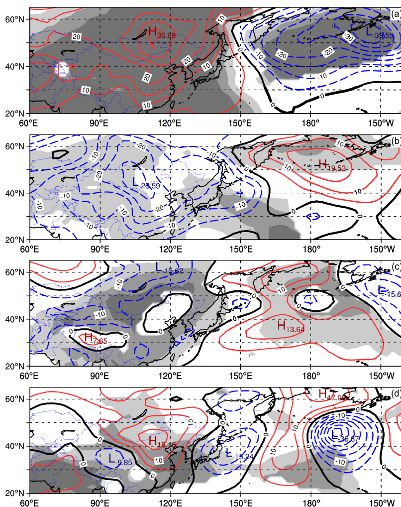
图 5 1948~2019 年东亚—西北太平洋海平面气压 (a) 瞬时维度为低值时、(b) 瞬时稳定度为低值时、(c) 瞬时维度为高值时、(d) 瞬时稳定度为高值时对应的海平面气压环流异常场 (单位: hPa) 的平均特征。红色实线、蓝色虚线、黑色粗实线分别表示正值、负值、零线, 等值线间隔是 5 hPa。灰色区域由浅到深分别代表有 60%、70% 和 80% 的指标成员在该区域有一致的信号分布
