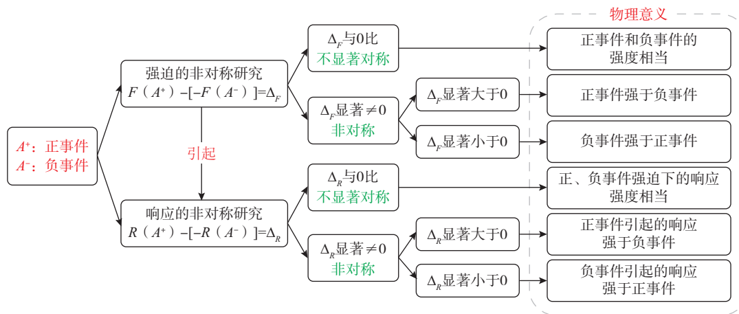
图2 非对称合成差分析方法
