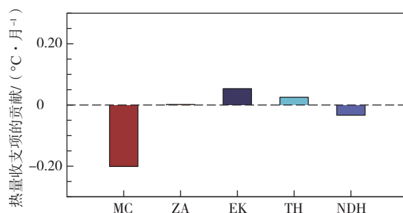
(b) La Niña 事件
