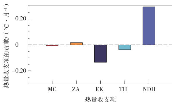
(c) El Niño 事件与 La Niña 事件的非对称合成差结果
