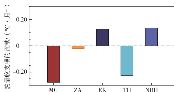
(a) El Niño 事件
