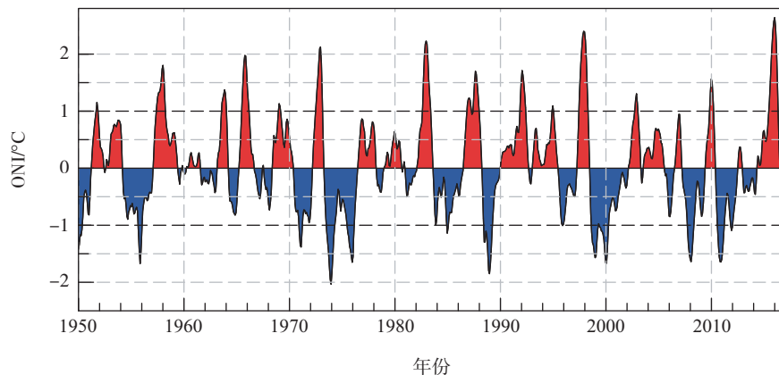
图 1 1950—2020 年 ONI 的时间序列
