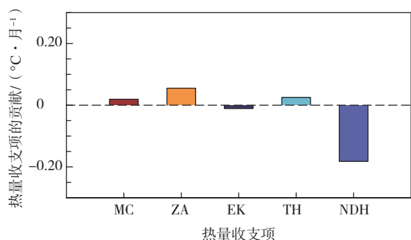
(c) El Niño 事件与 La Niña 事件的非对称合成差结果
