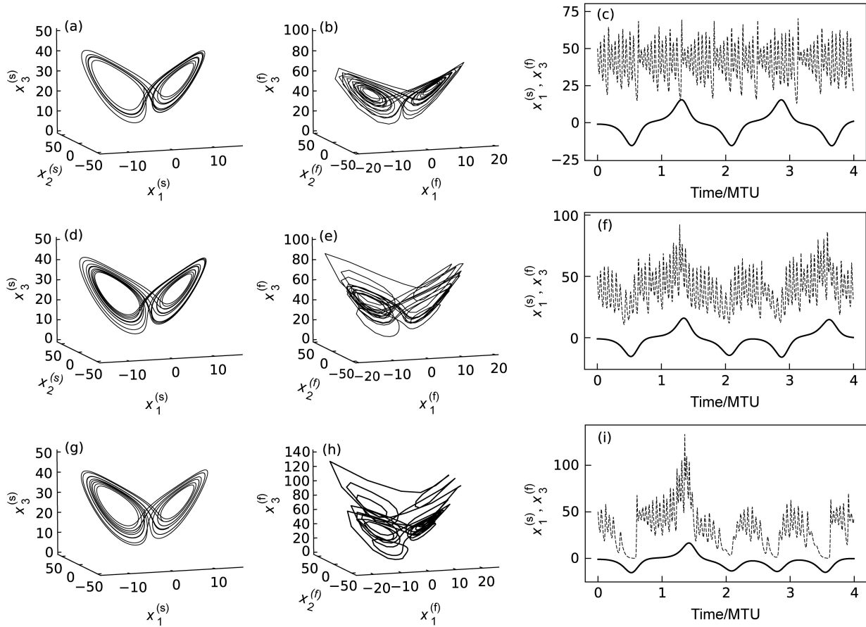
图1 不同耦合强度时慢(左)、快(中)系统三维运动轨迹和 x_1^{(s)} (实线)、 x_3^{(f)} (虚线)随时间 t [单位: MTU (model time units)]演变的时间序列(右): (a-c) \varepsilon_s=0, \varepsilon_f=0 ; (d-f) \varepsilon_s=10^{-2}, \varepsilon_f=10 ; (g-i) \varepsilon_s=10^{-1.8}, \varepsilon_f=24 . \varepsilon_s ( \varepsilon_f ) 为慢(快)系统中控制耦合强度的参数。
