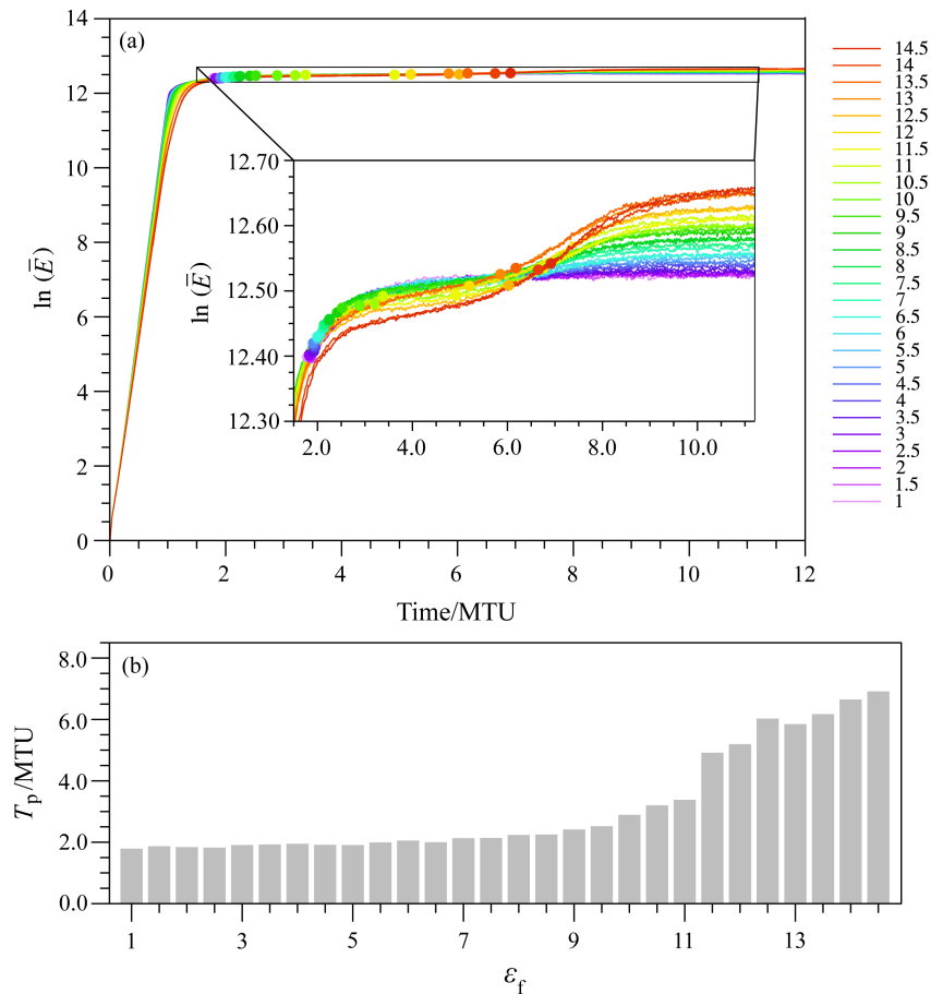
图3 在 \epsilon_s=10^{-2} 时, 取不同 \epsilon_f 值时快系统 (a) 相对误差的自然对数随时间增长曲线和 (b) 可预报时间 ( T_p ) 随 \epsilon_f 的变化。
