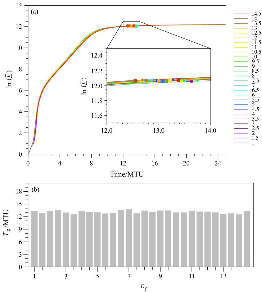
图6 在 \epsilon_s=10^{-2} 时, 取不同 \epsilon_f 值时慢系统 (a) 相对误差的自然对数随时间增长曲线和 (b) 可预报时间 ( T_p ) 随 \epsilon_f 的变化。
