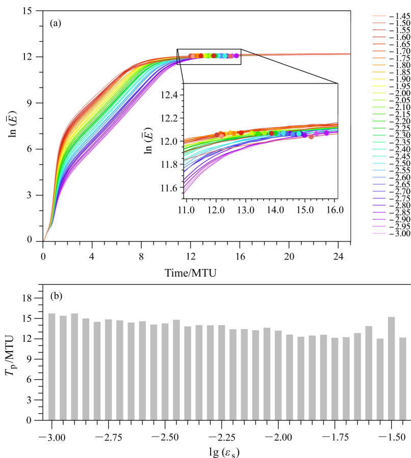
图5 在 \varepsilon_f=12 时, 取不同 \varepsilon_s 值时慢系统 (a) 相对误差的自然对数随时间增长曲线和 (b) 可预报时间 ( T_p ) 随 \varepsilon_s 的变化。
