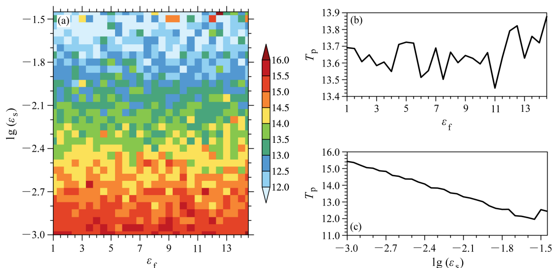
图7 (a) 不同耦合强度时, 慢系统的可预报时间 (单位: MTU); (b) 对图 a 沿 \epsilon_s 轴平均后, 慢系统可预报时间随 \epsilon_f 的变化和 (c) 对图 a 沿 \epsilon_f 轴平均后, 慢系统可预报时间随 \epsilon_s 的变化。 \epsilon_s 值的大小均以对数化后的 \lg(\epsilon_s) 表示。
