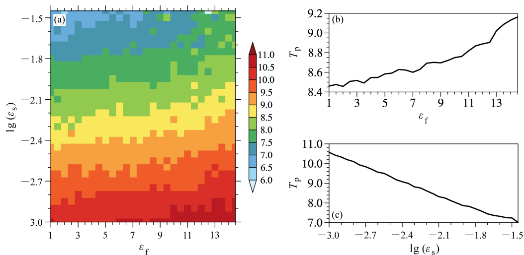
图8 (a) 不同耦合强度时, 耦合系统整体的可预报时间 (单位: MTU); (b) 对图 a 沿 \epsilon_s 轴平均后, 快系统可预报时间随 \epsilon_f 的变化和 (c) 对图 a 沿 \epsilon_f 轴平均后, 整体可预报时间随 \epsilon_s 的变化。 \epsilon_s 值的大小均以对数化后的 \lg(\epsilon_s) 表示。
