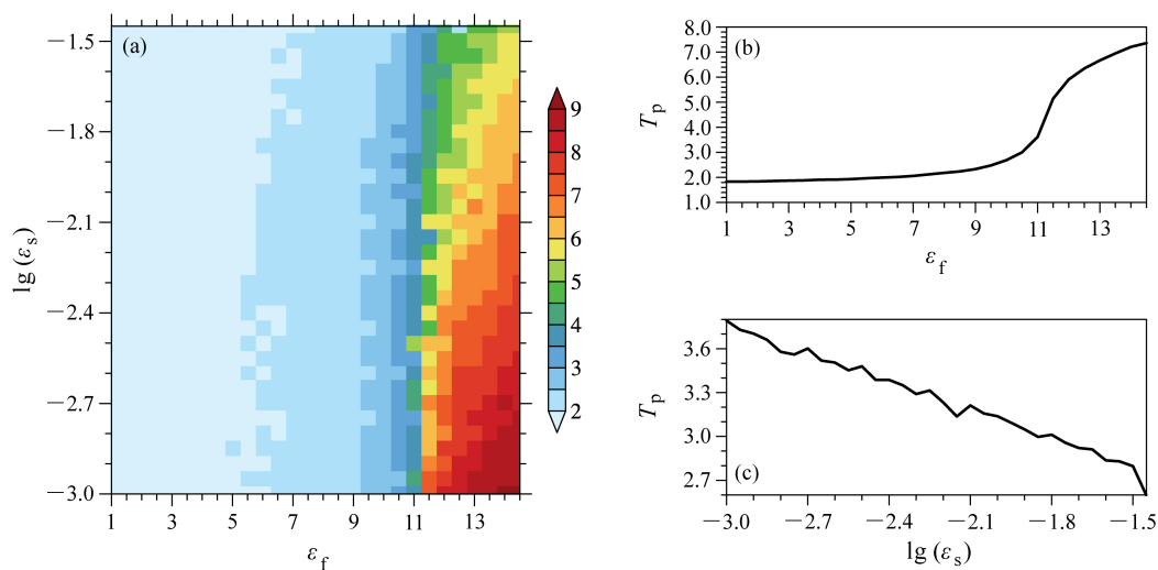
图4 (a) 不同耦合强度时, 快系统的可预报时间 (单位: MTU); (b) 对图 a 沿 \varepsilon_s 轴平均后, 快系统可预报时间随 \varepsilon_f 的变化和 (c) 对图 a 沿 \varepsilon_f 轴平均后, 快系统可预报时间随 \varepsilon_s 的变化。 \varepsilon_s 值的大小均以对数化后的 \lg(\varepsilon_s) 表示。
