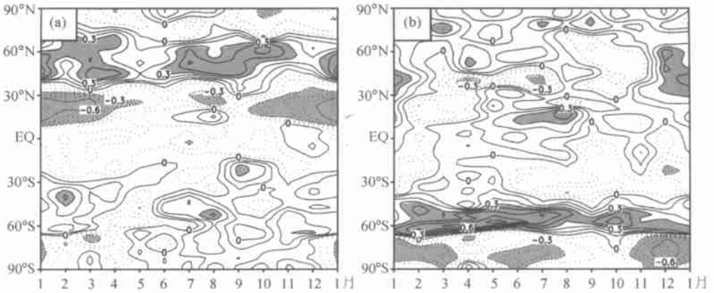
图 4 涛动指数与纬向平均 1000 hPa 温度场的相关系数随季节和纬度的变化图，其余同图 2
