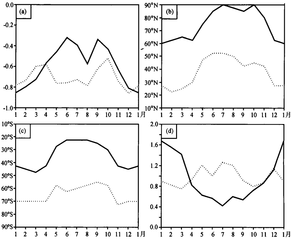
图1 (a) 北半球(实线)和南半球(虚线)纬向平均的月平均SIP场之间求纬向相关所得的最大负相关系数的年变化曲线 (b) 北半球上述最大负相关系数相对应的两个纬度值的年变化曲线(较高纬度为实线, 较低纬度为虚线); (c) 与(b)相似, 但为南半球的情况; (d) I_{AO} (实线) 和 I_{AAO} (虚线) 的标准差的年变化曲线图
