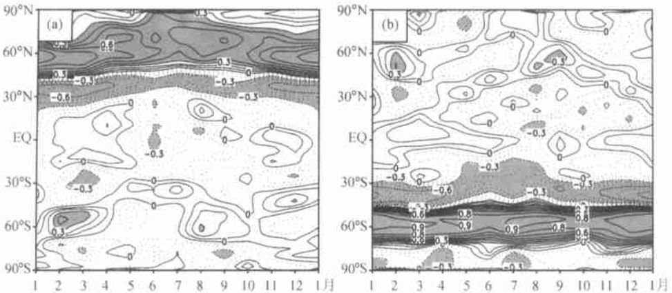
图 3 涛动指数与纬向平均的月平均 500 hPa 为纬向风场的相关系数随季节和纬度的变化图，其余同图 2
