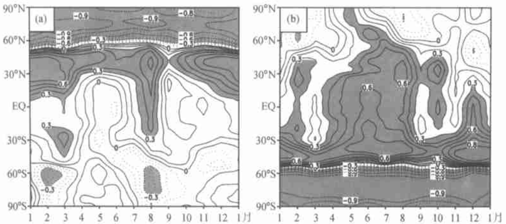
图2 涛动指数与纬向平均的海平面气压场相关系数随季节和纬度的变化曲线图 阴影区为通过95%的置信检验, 实线为正相关, 虚线为负相关. (a) I_{AG} (b) I_{AAO}
