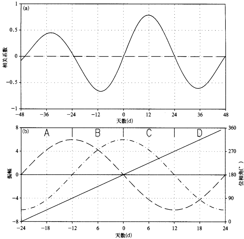
图 5 P_{C1} 和 P_{C2} 之间超前和滞后相关系数变化和基于 48 d 振荡周期 MJO 的位相分类示意图 (a. P_{C1} 与 P_{C2} 超前和滞后相关系数时间变化, b. MJO 的 A, B, C 和 D 位相对应的 P_{C1} (虚线)、 P_{C2} (点虚线) 和位相角 (实线) 时间变化。左侧坐标轴表示 P_{C1} 和 P_{C2} 振幅,右侧坐标表示位相角度(单位:度)
