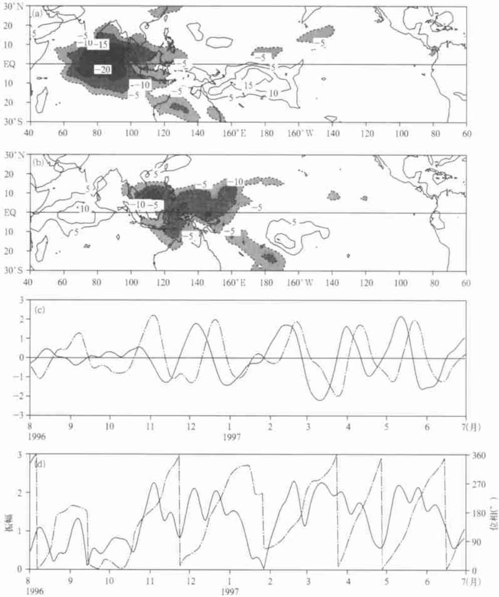
图 2 1996 年 8 月至 1997 年 6 月期间经过 20~120 带通滤波之后的 OLR 场 EOF 分析结果 (a. EOF1, b. EOF2, 等值线间隔 5 \text{ W/m}^2 , 阴影区表示负值区, c. EOF1 和 EOF2 对应的时间系数 P_{C_1} (实线) 和 P_{C_2} (虚线) 变化, d. 位相角 (虚线, 右侧坐标轴) 和振幅 A (实线, 左侧坐标轴) 时间变化)
